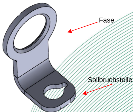
Bild 4: Anschlagpunkt, Typ: TS-Lasche (TS-011) (mit Sollbruchstelle, mit Fasen (1 x 45°))
