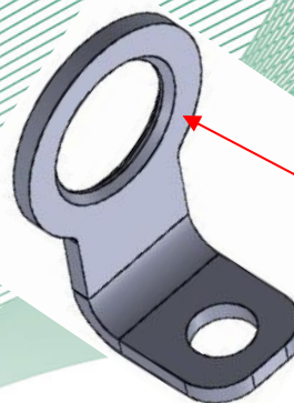
Bild 3: Anschlagpunkt, Typ: TS-Lasche (TS-011) (ohne Sollbruchstelle, mit Fasen (2 x 45°))
